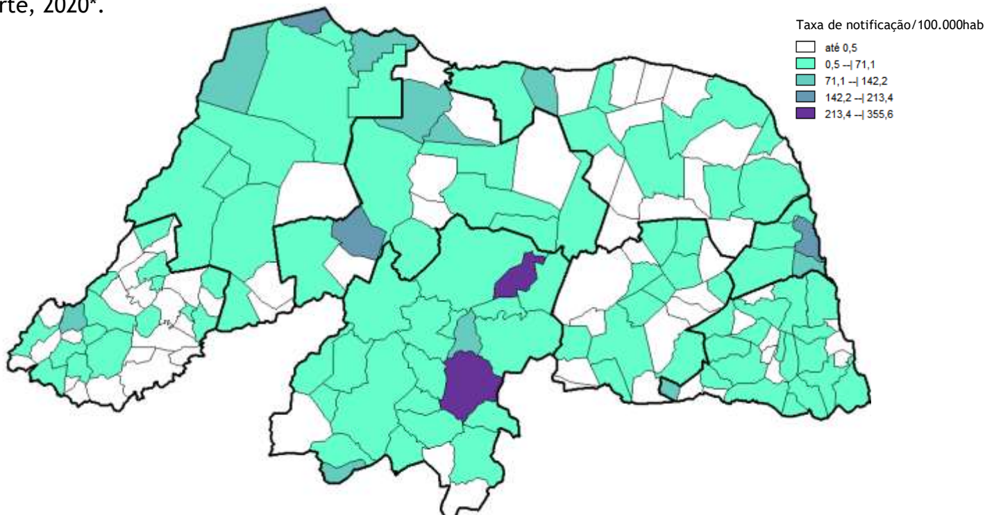
Figura 1 - Taxa de notificação (casos/100.000hab) por município de residência, Rio Grande do Norte, 2020*.
