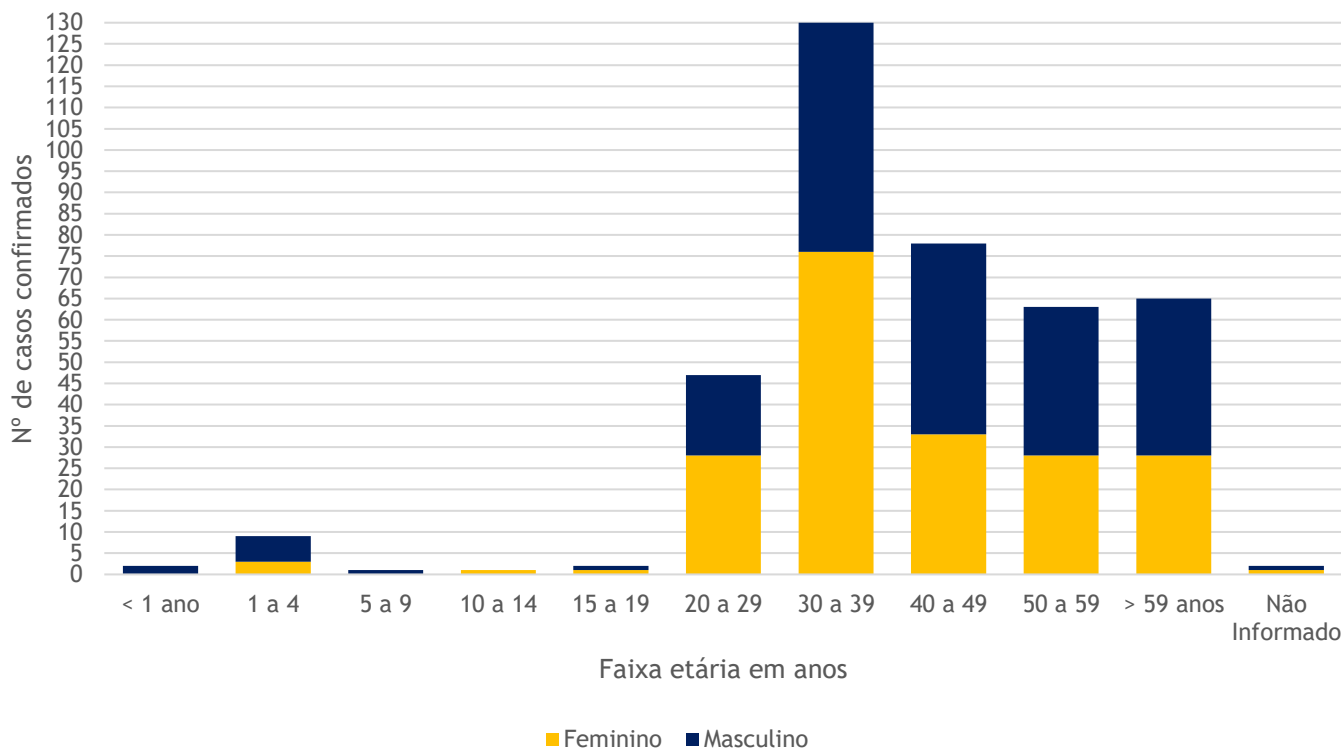
Gráfico 3 - Casos confirmados por COVID-19 de acordo com faixa etária e sexo, Rio Grande do Norte, 2020*.
