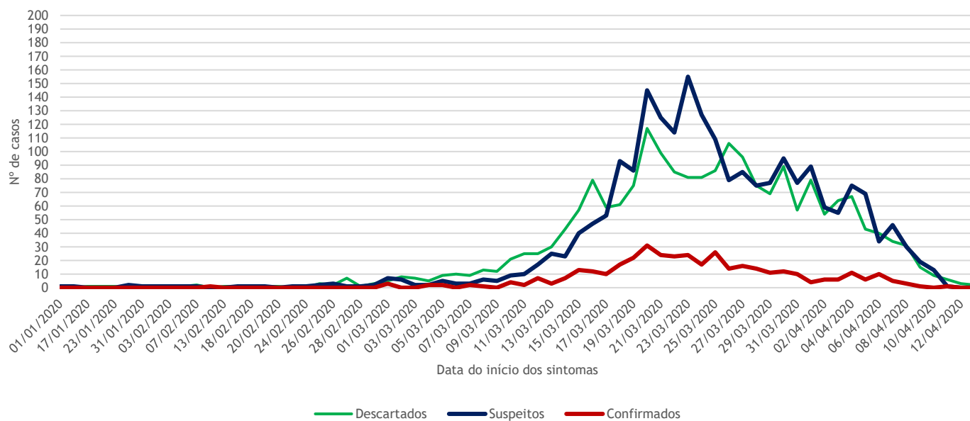
Gráfico 2 - Casos Notificados por COVID-19 de acordo com a data de início de sintomas informada e status de evolução, Rio Grande do Norte, 2020*.
